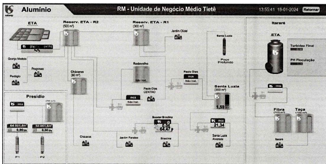
Figura 1 – Croqui do setor de abastecimento presente no Município de Alumínio
